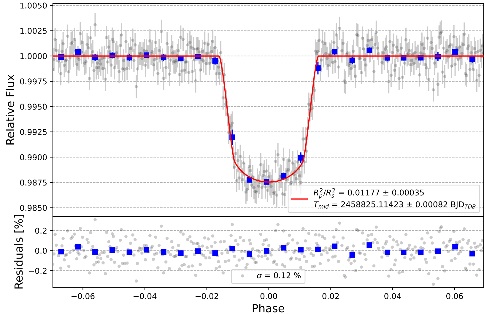
XO-6 b
