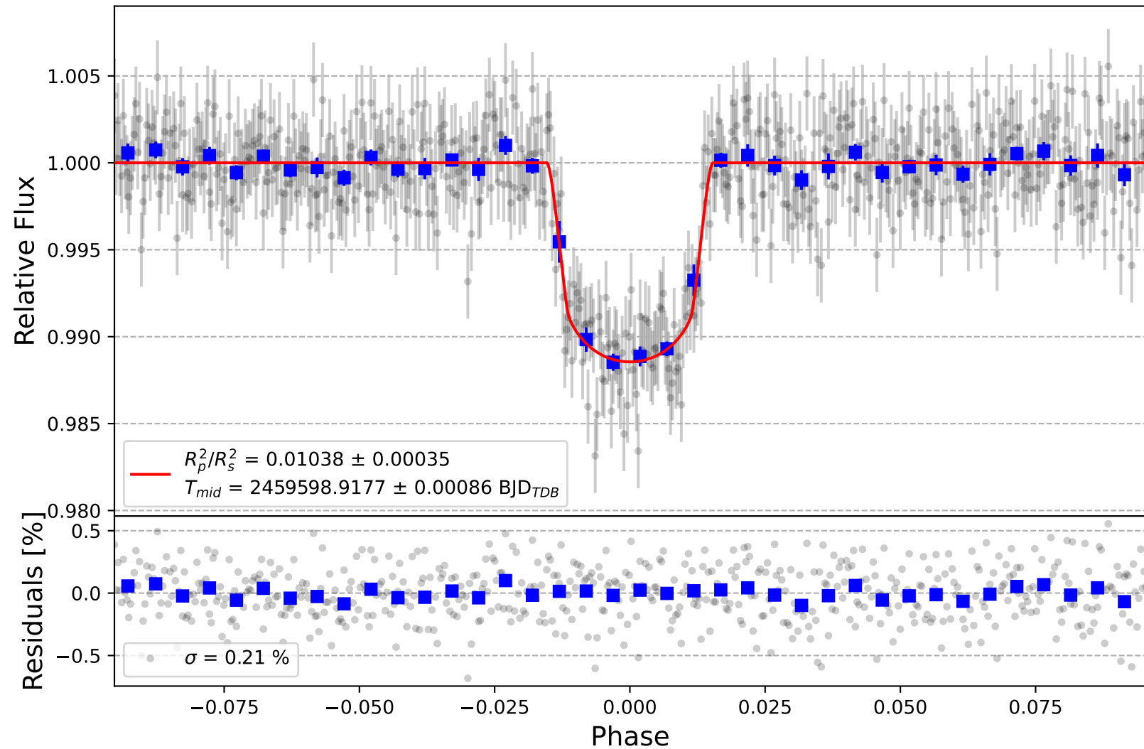
XO-5 b
