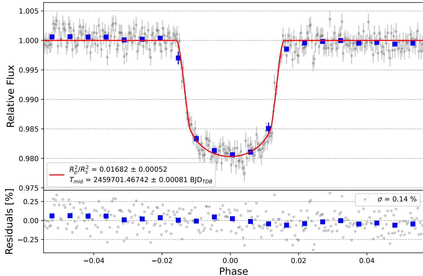
XO-1 b
