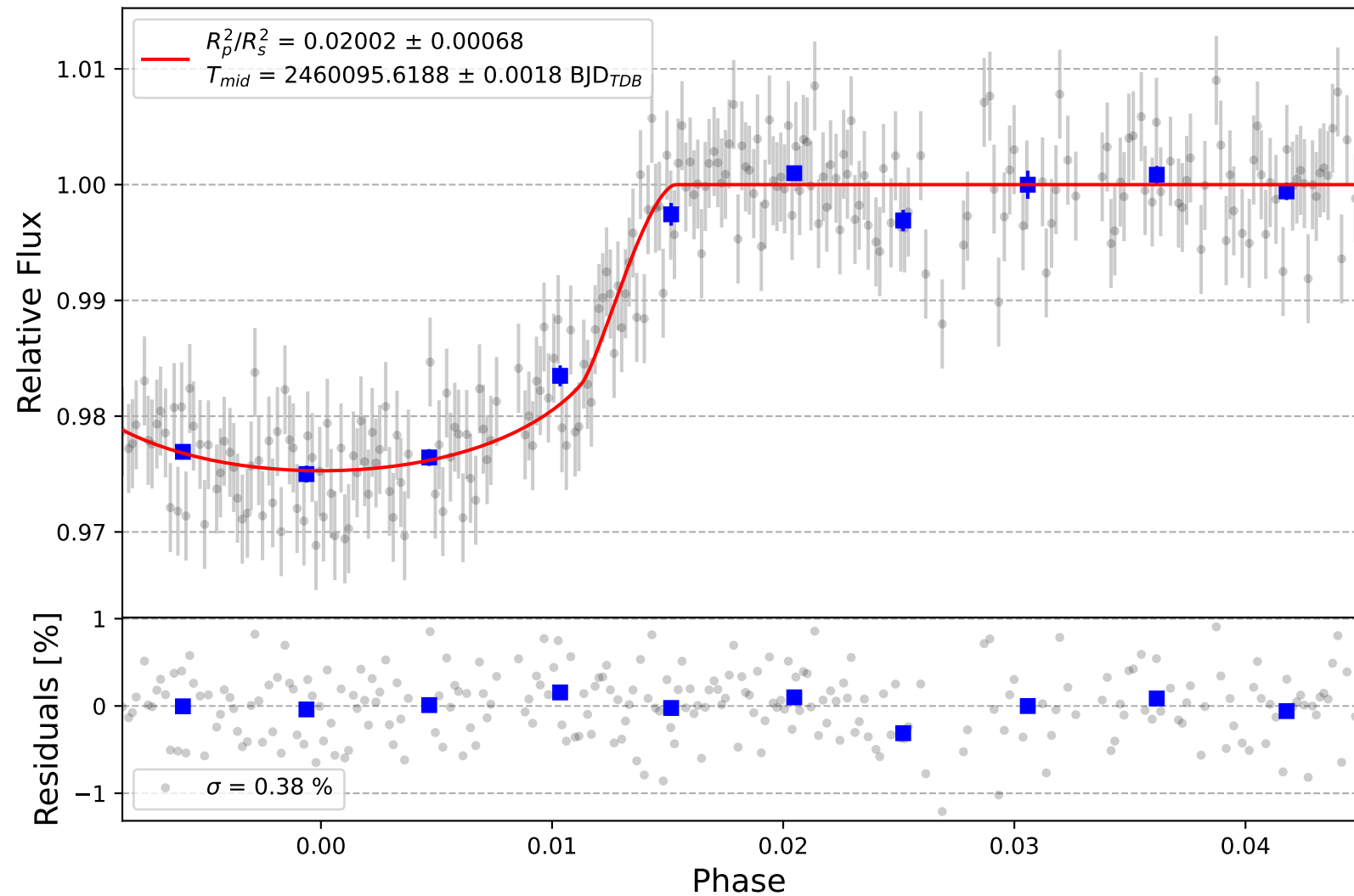
XO-1 b
