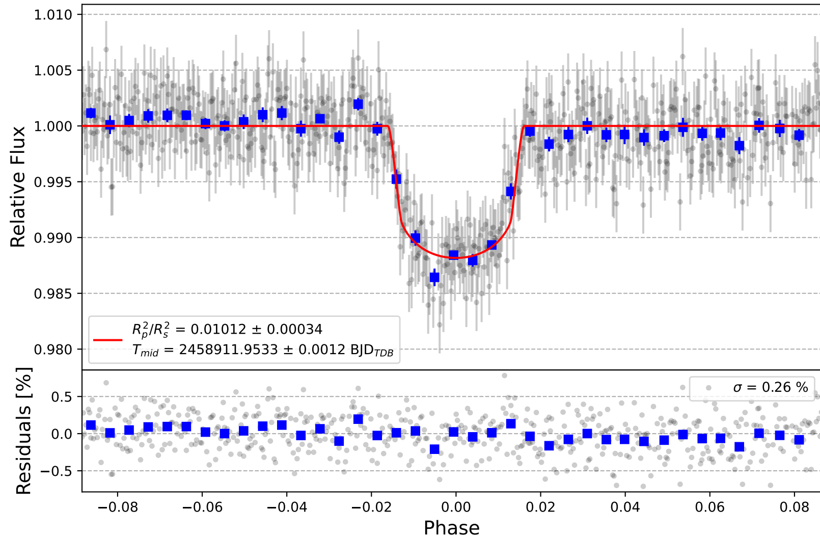
WASP-56 b
