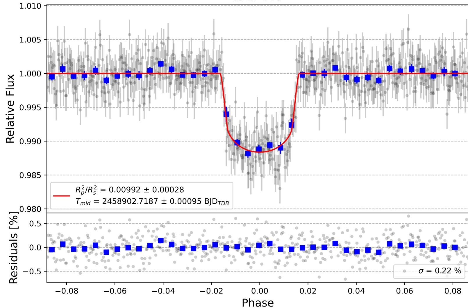
WASP-56 b
