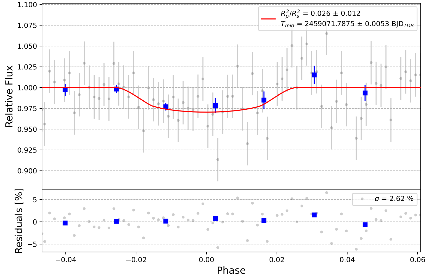
TrES-5 b
