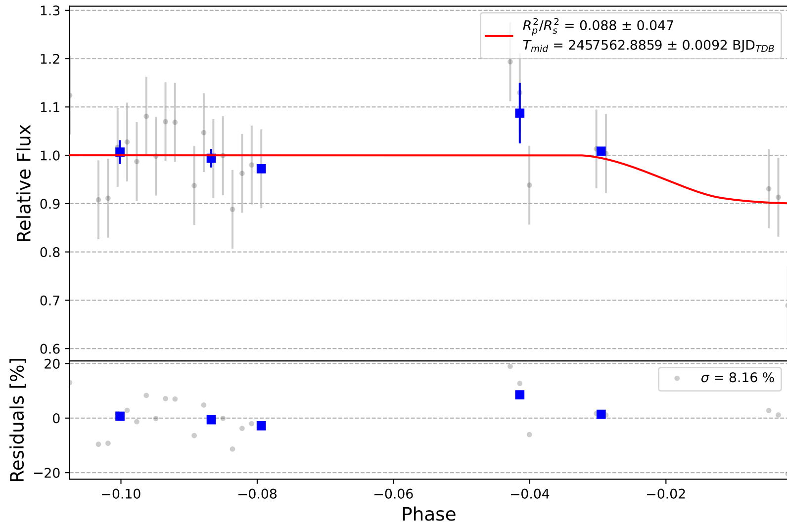
TrES-5 b
