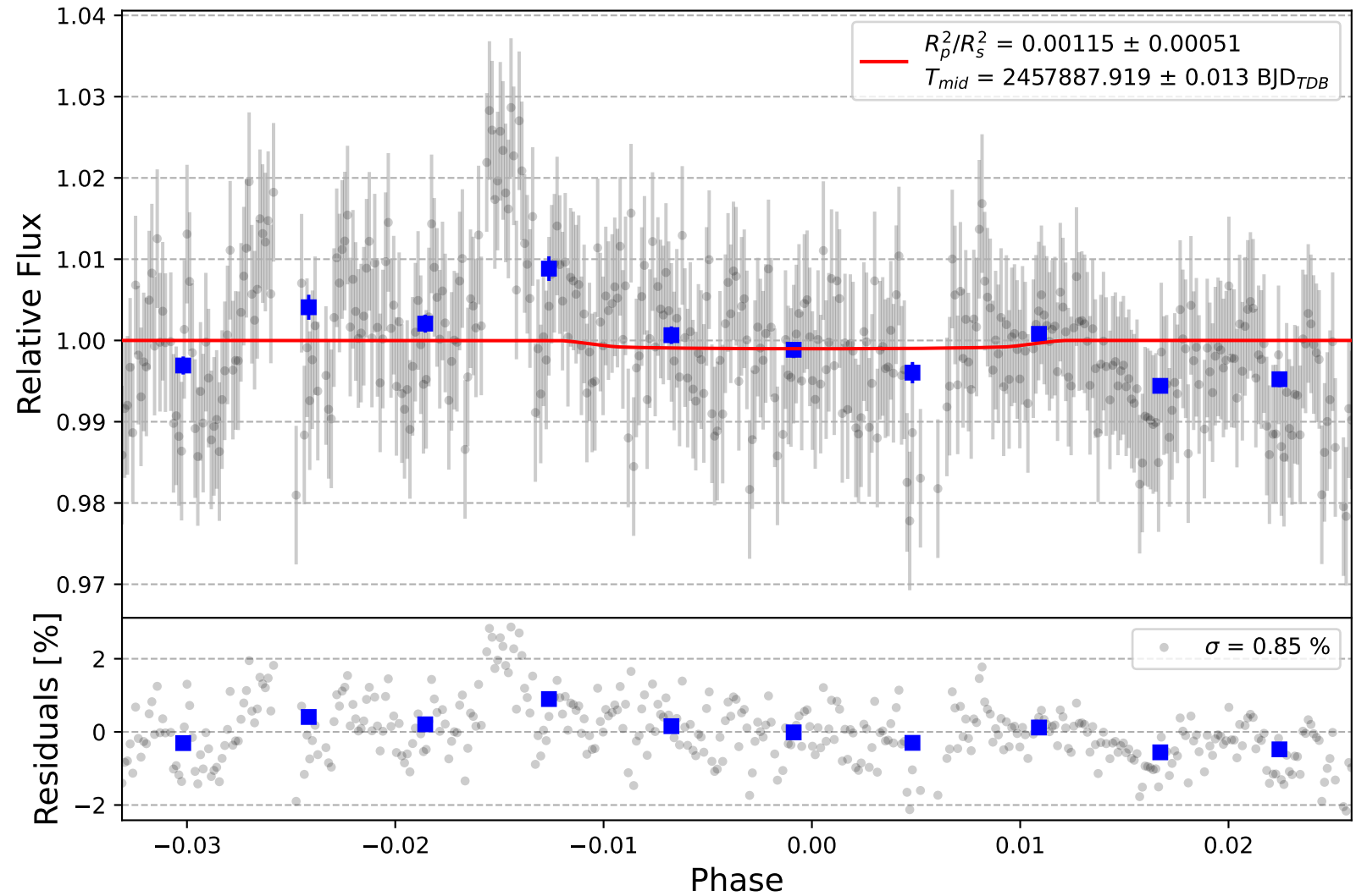
TrES-4 b
