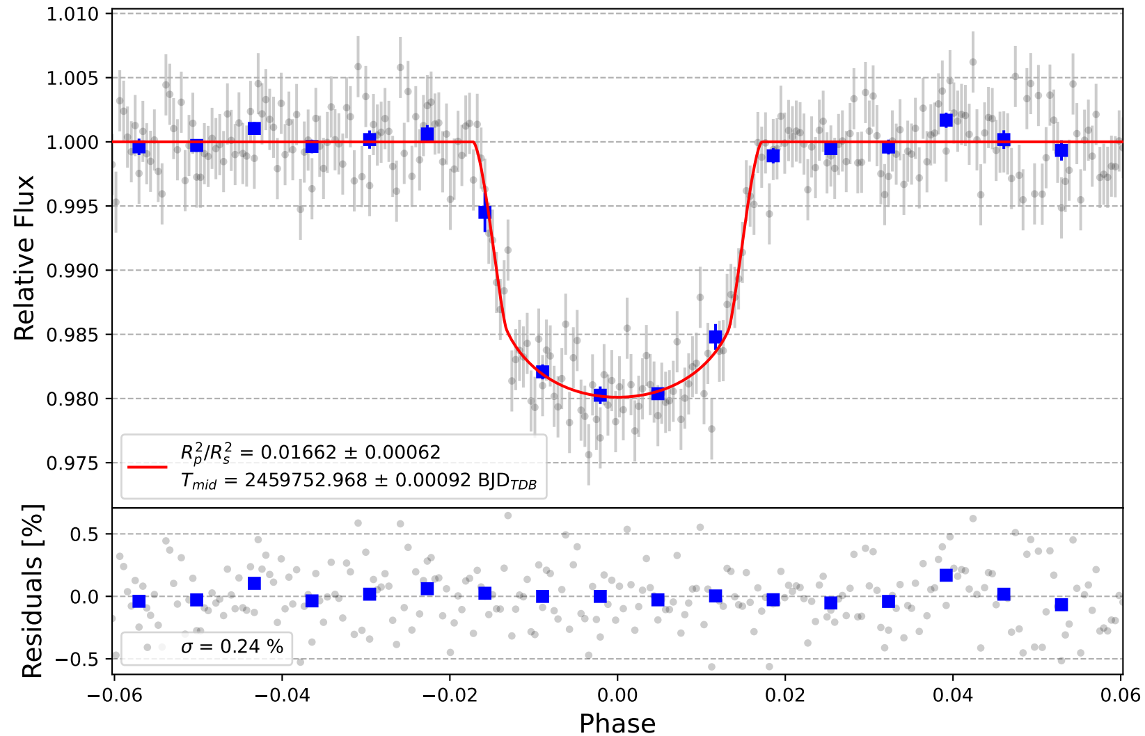
TrES-1 b
