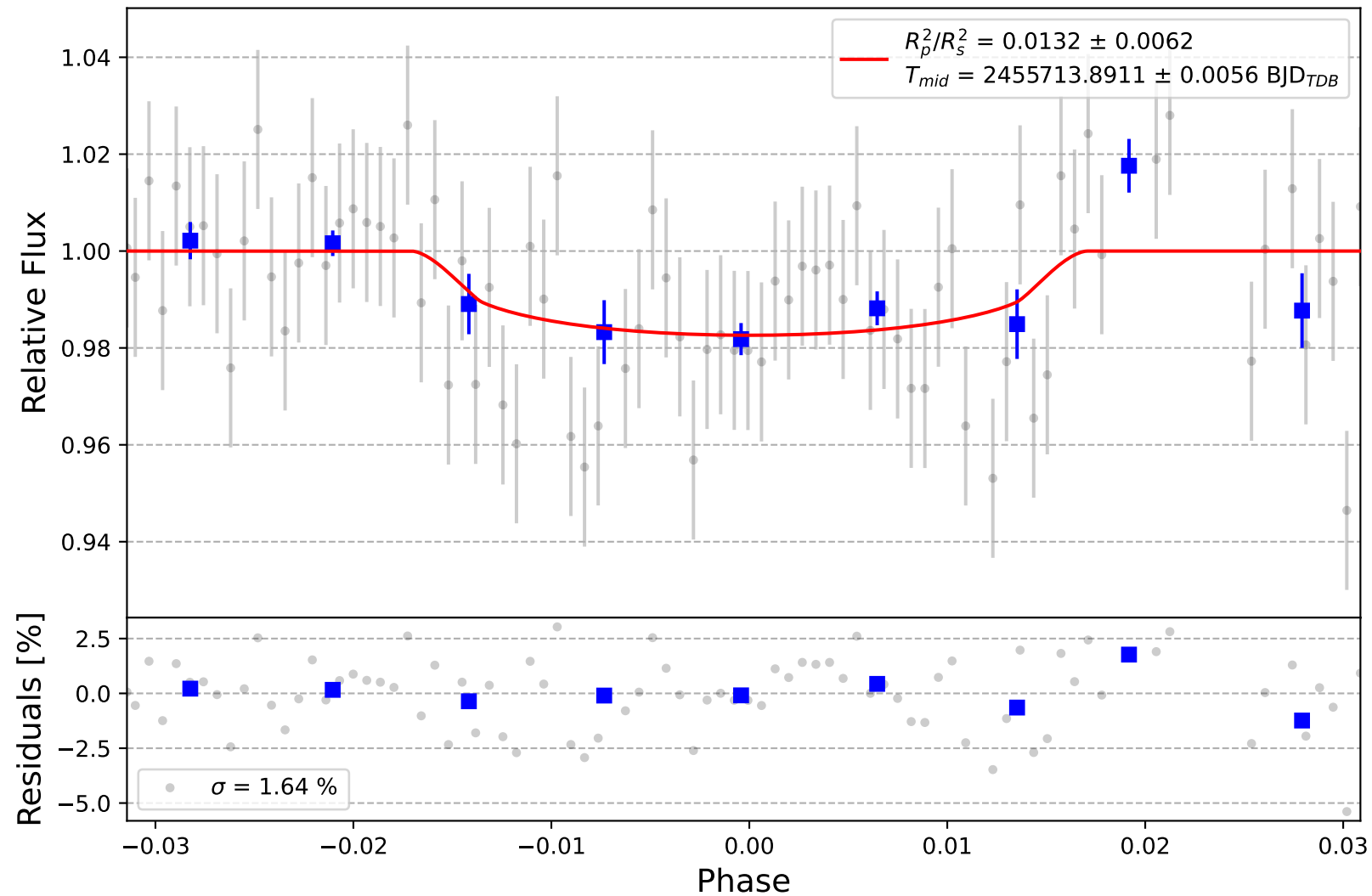
TrES-1 b
