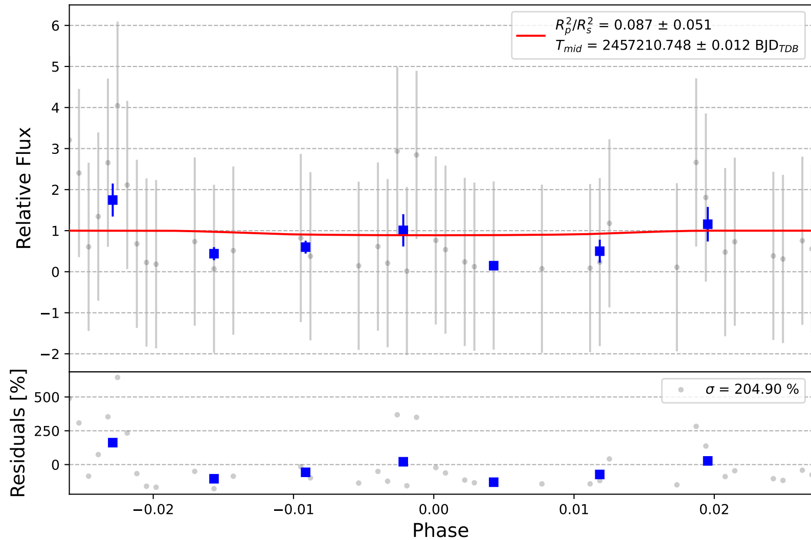
TrES-1 b
