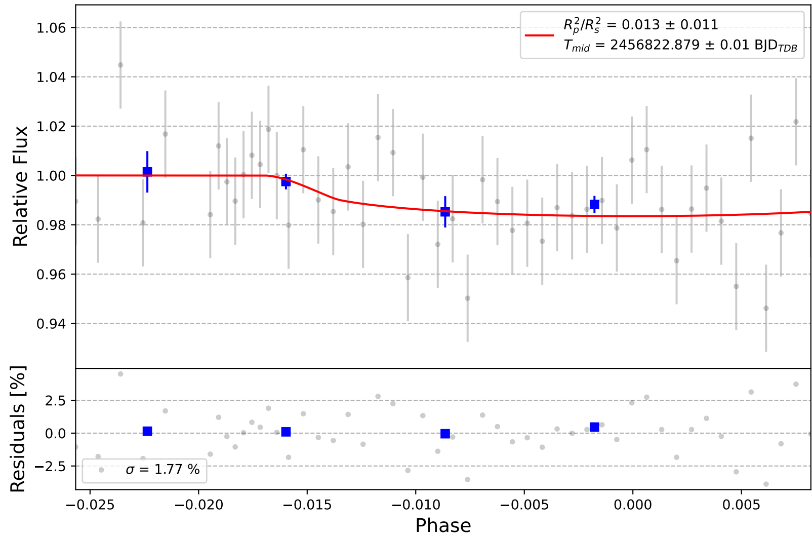
TrES-1 b
