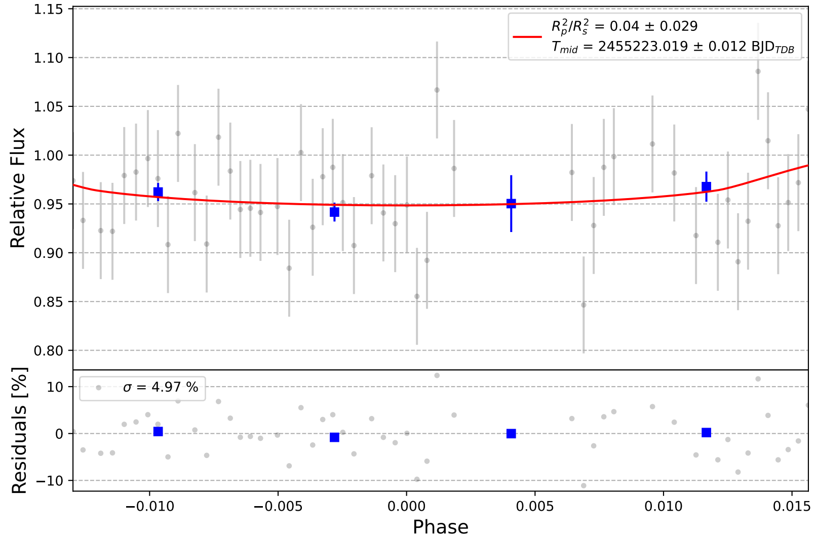
TrES-1 b
