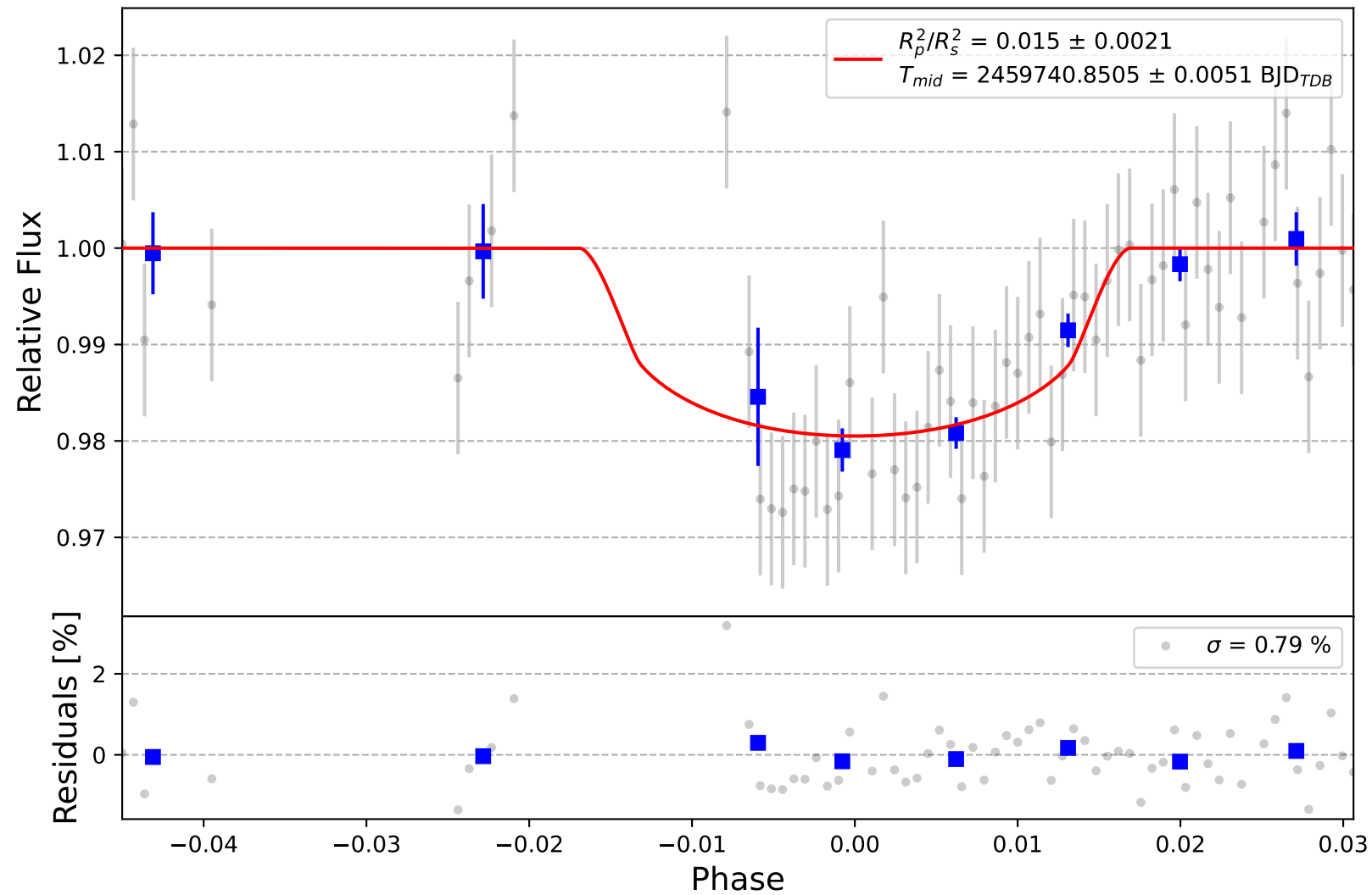
TrES-1 b
