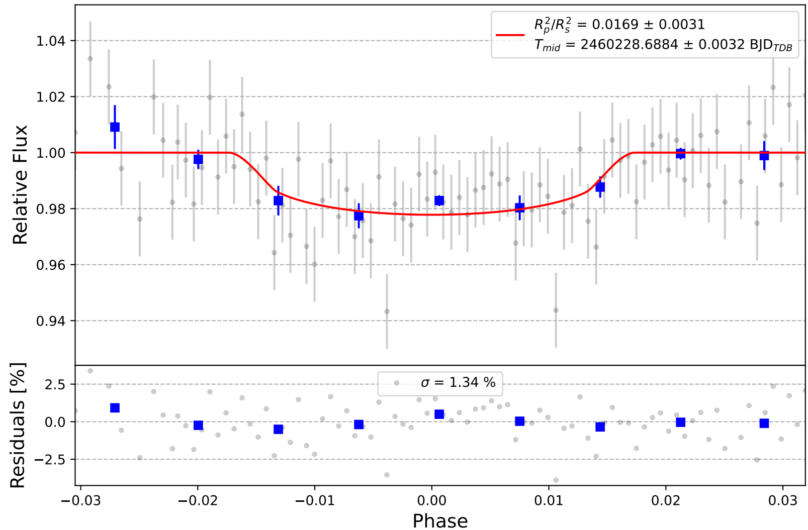
TrES-1 b
