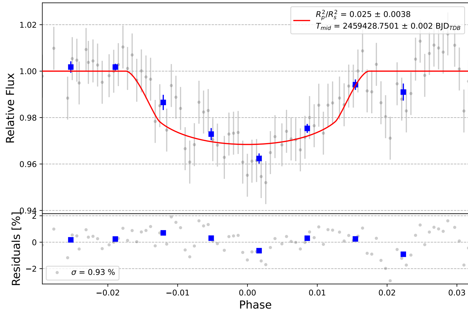
TrES-1 b
