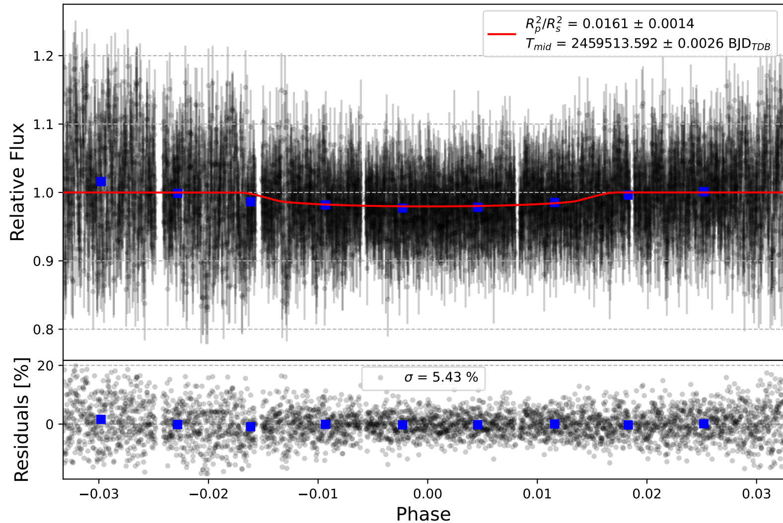
TrES-1 b
