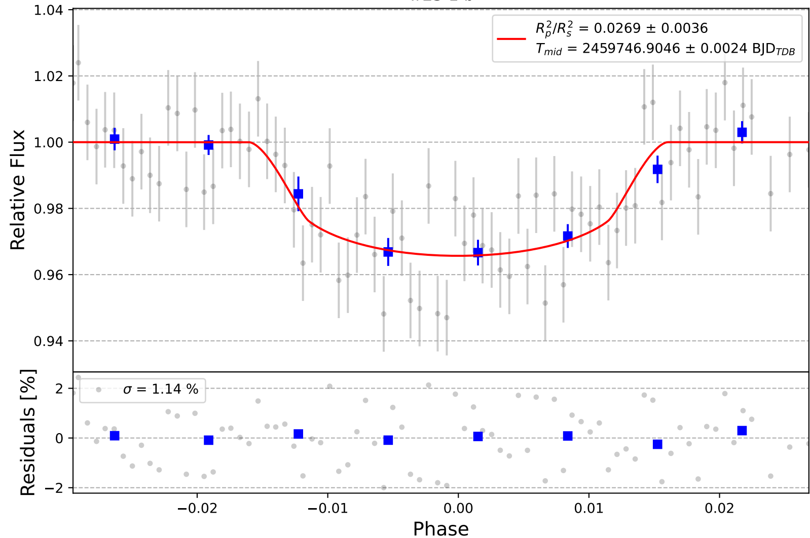
TrES-1 b
