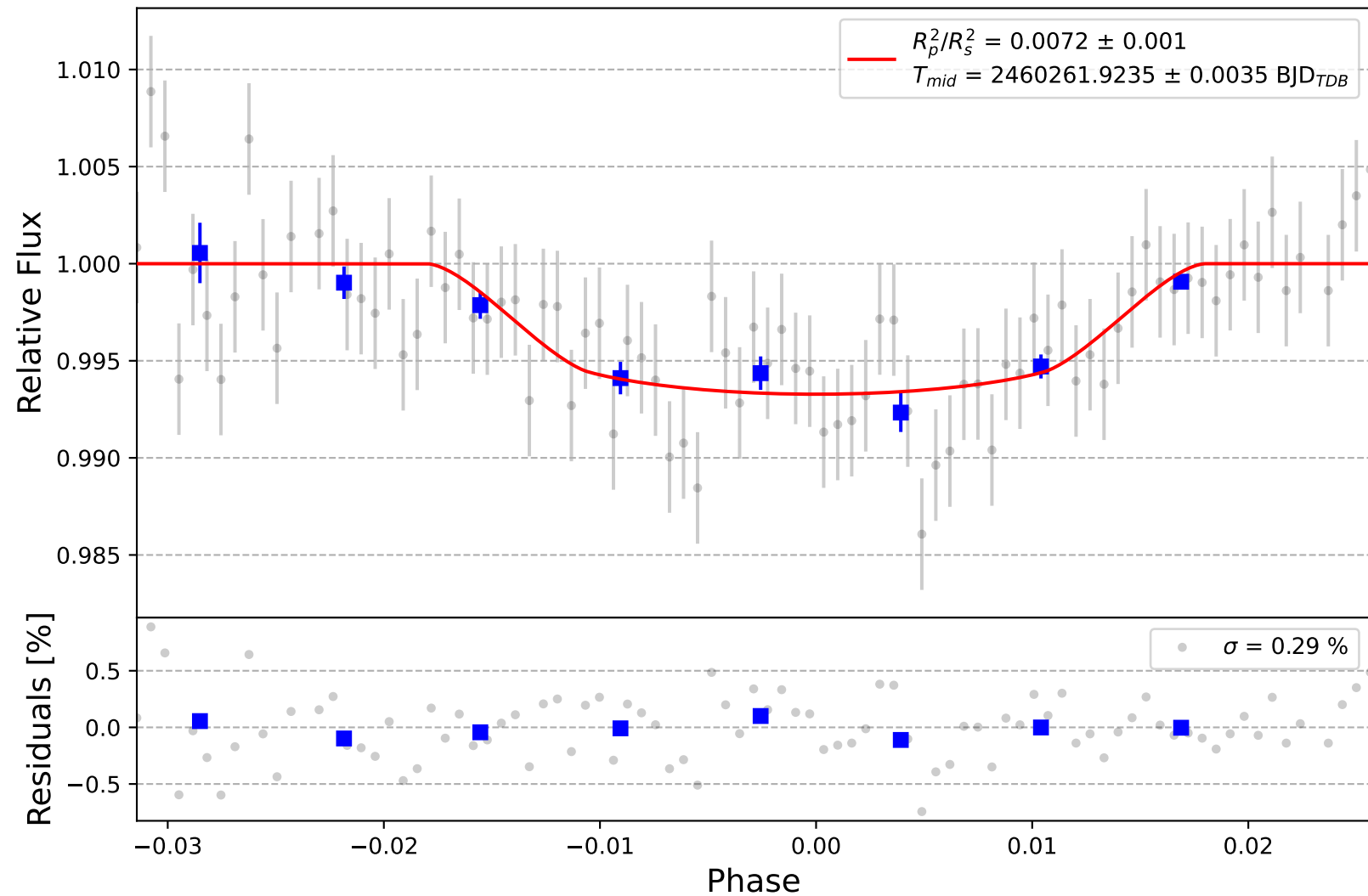
TOI-3819 b
