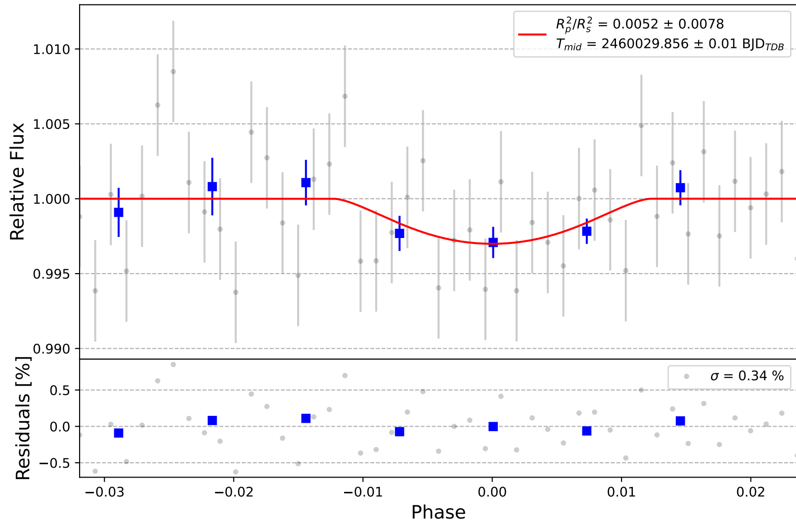
TOI-3807 b
