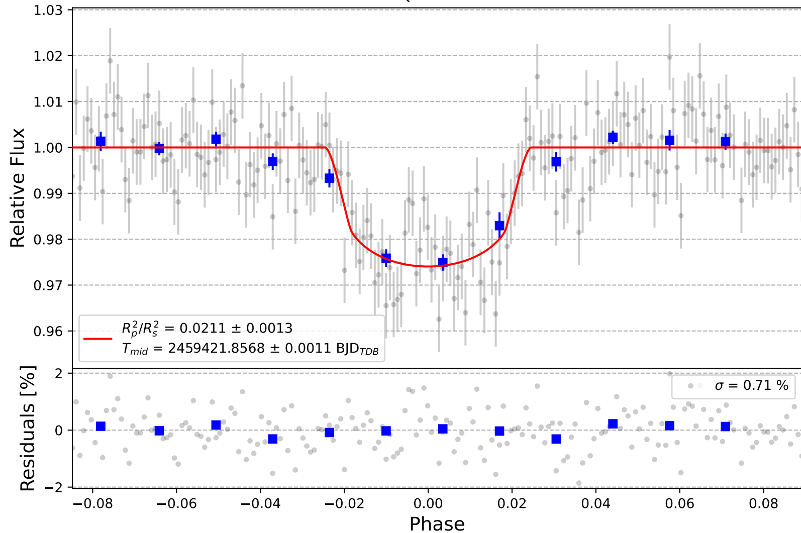
Qatar-9 b
