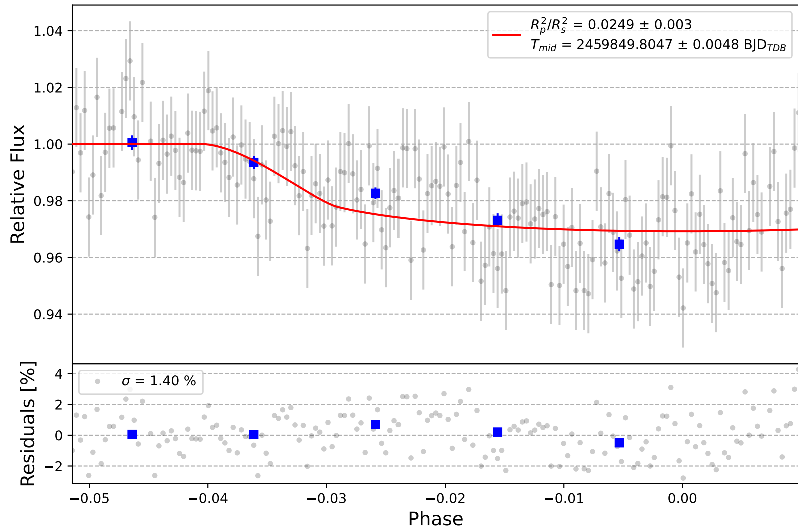
Qatar-7 b
