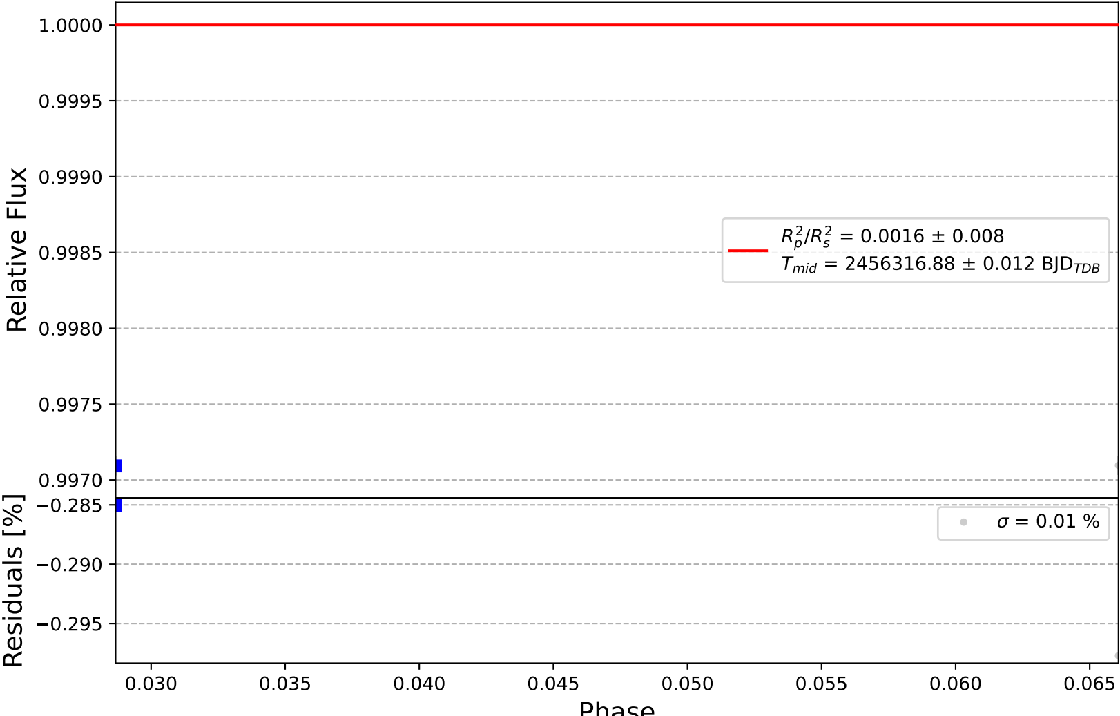
Qatar-2 b
