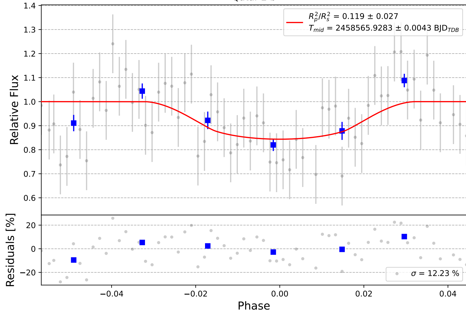
Qatar-2 b
