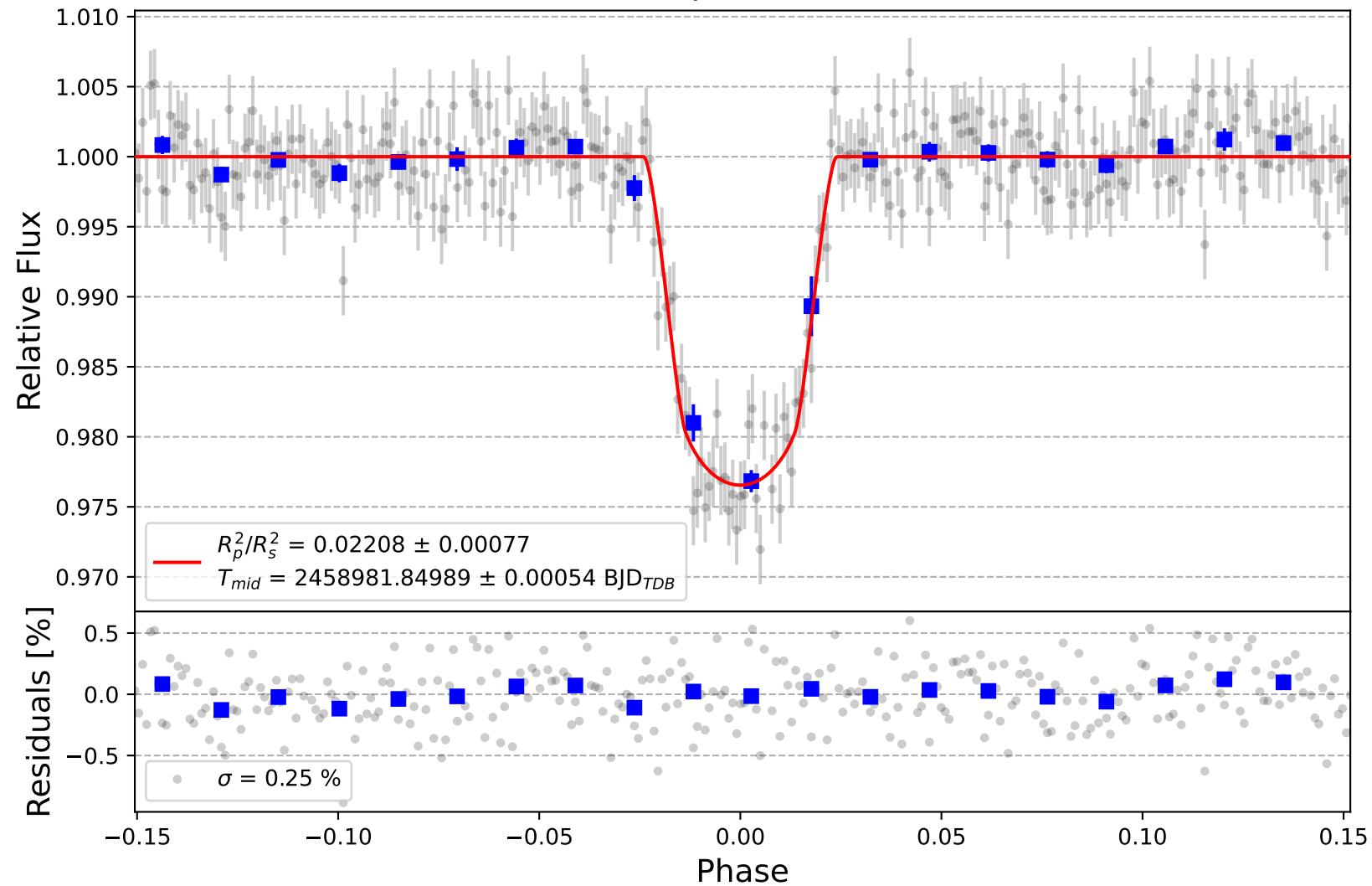
Qatar-1 b
