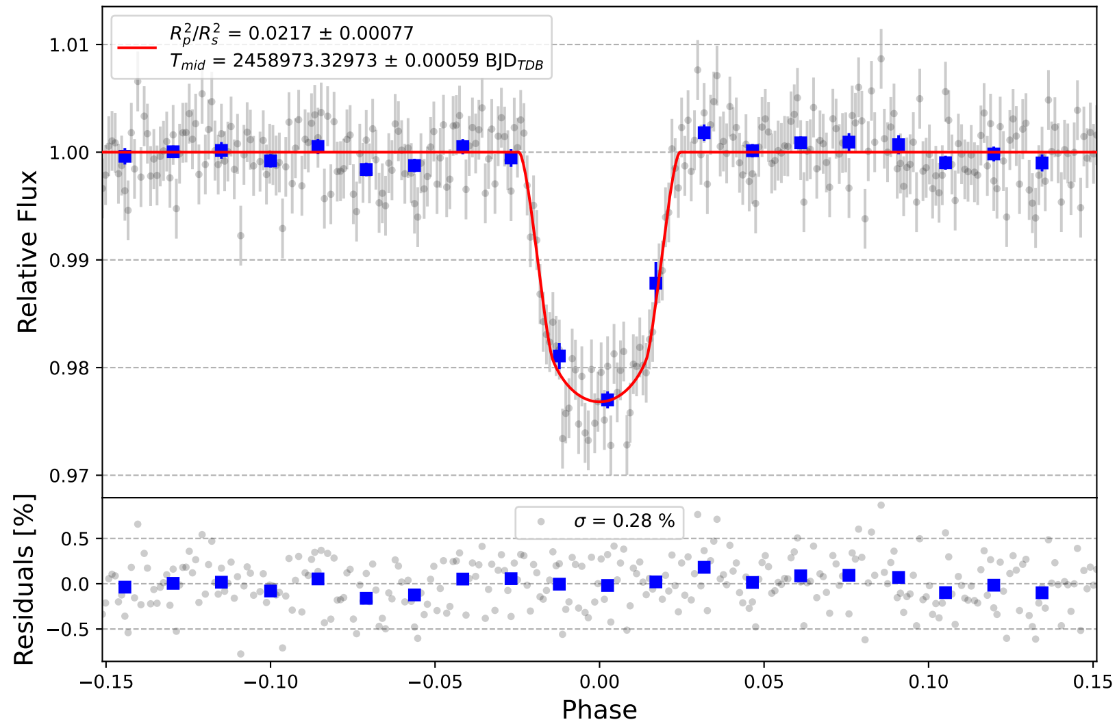
Qatar-1 b
