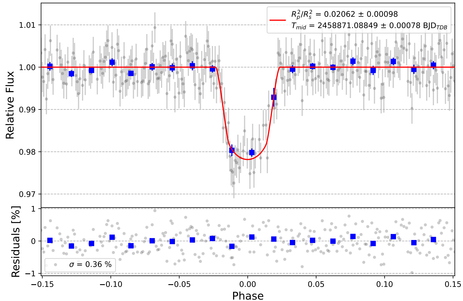
Qatar-1 b
