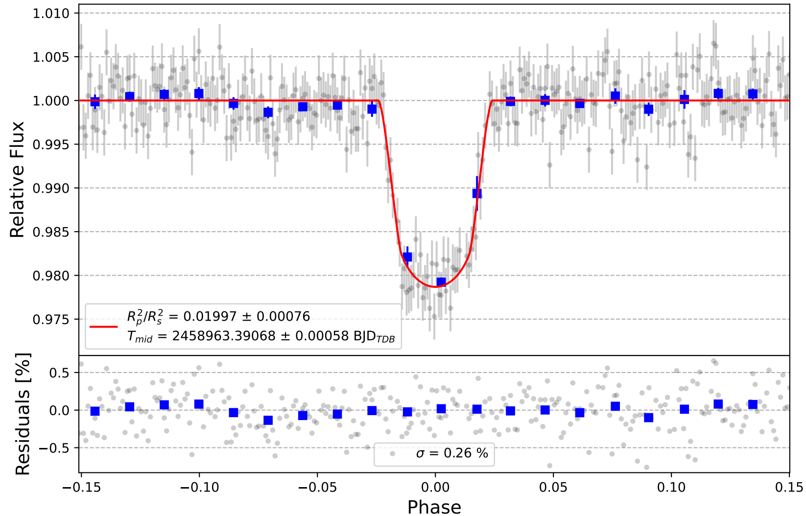
Qatar-1 b
