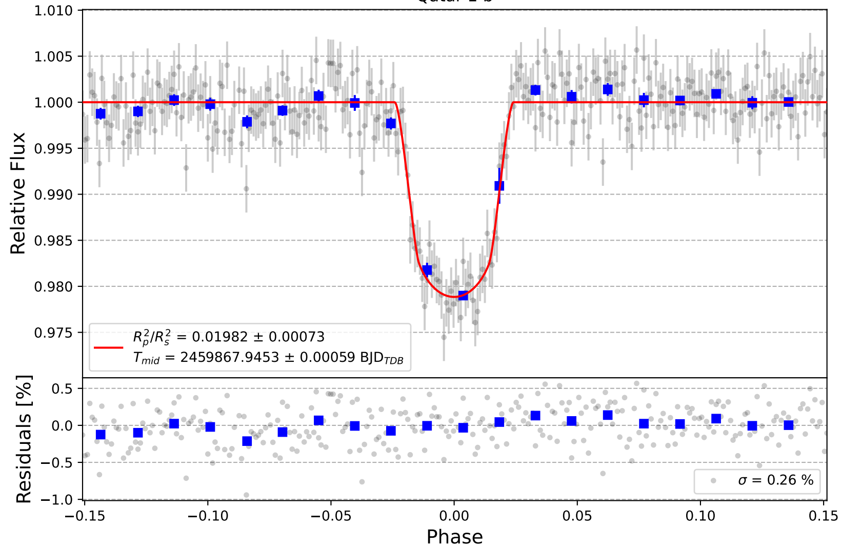
Qatar-1 b
