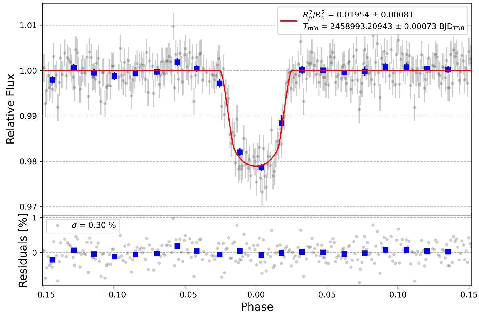
Qatar-1 b
