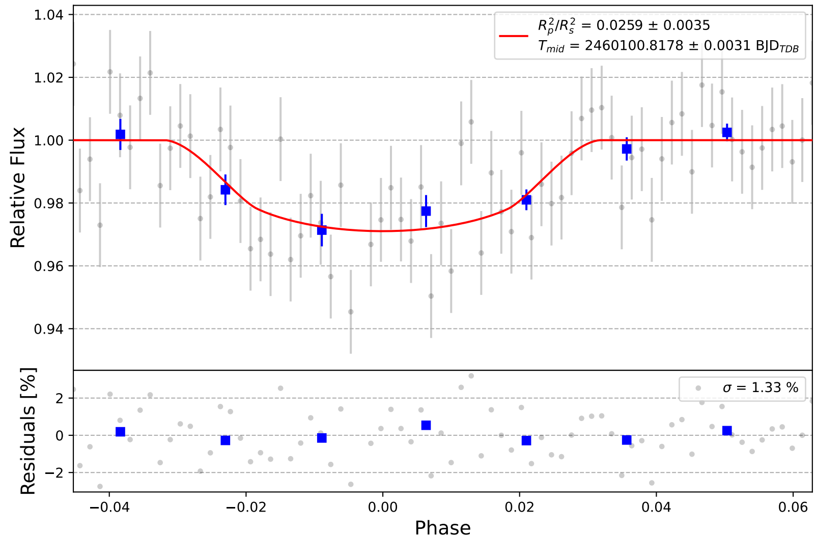
Qatar-1 b
