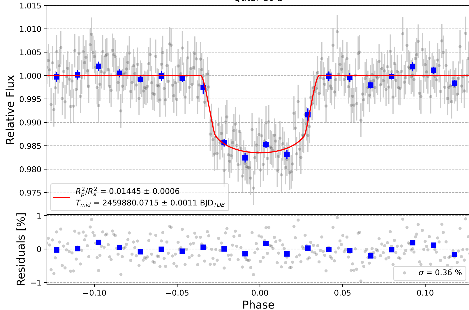
Qatar-10 b
