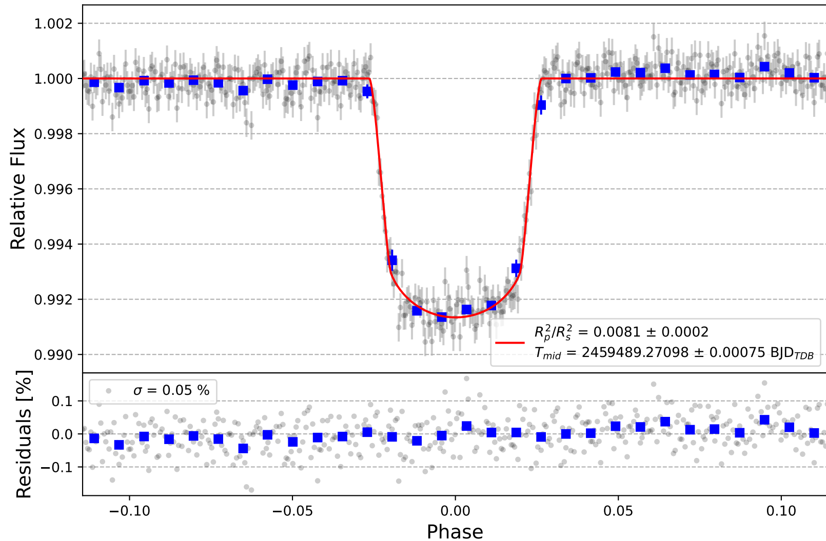
KELT-7 b
