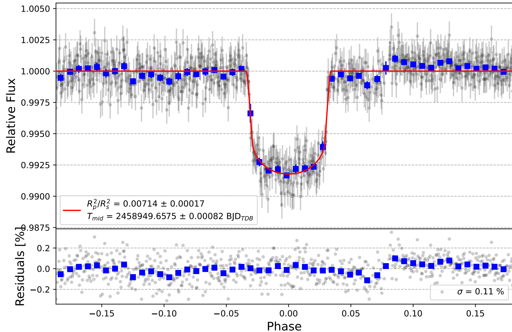
KELT-18 b
