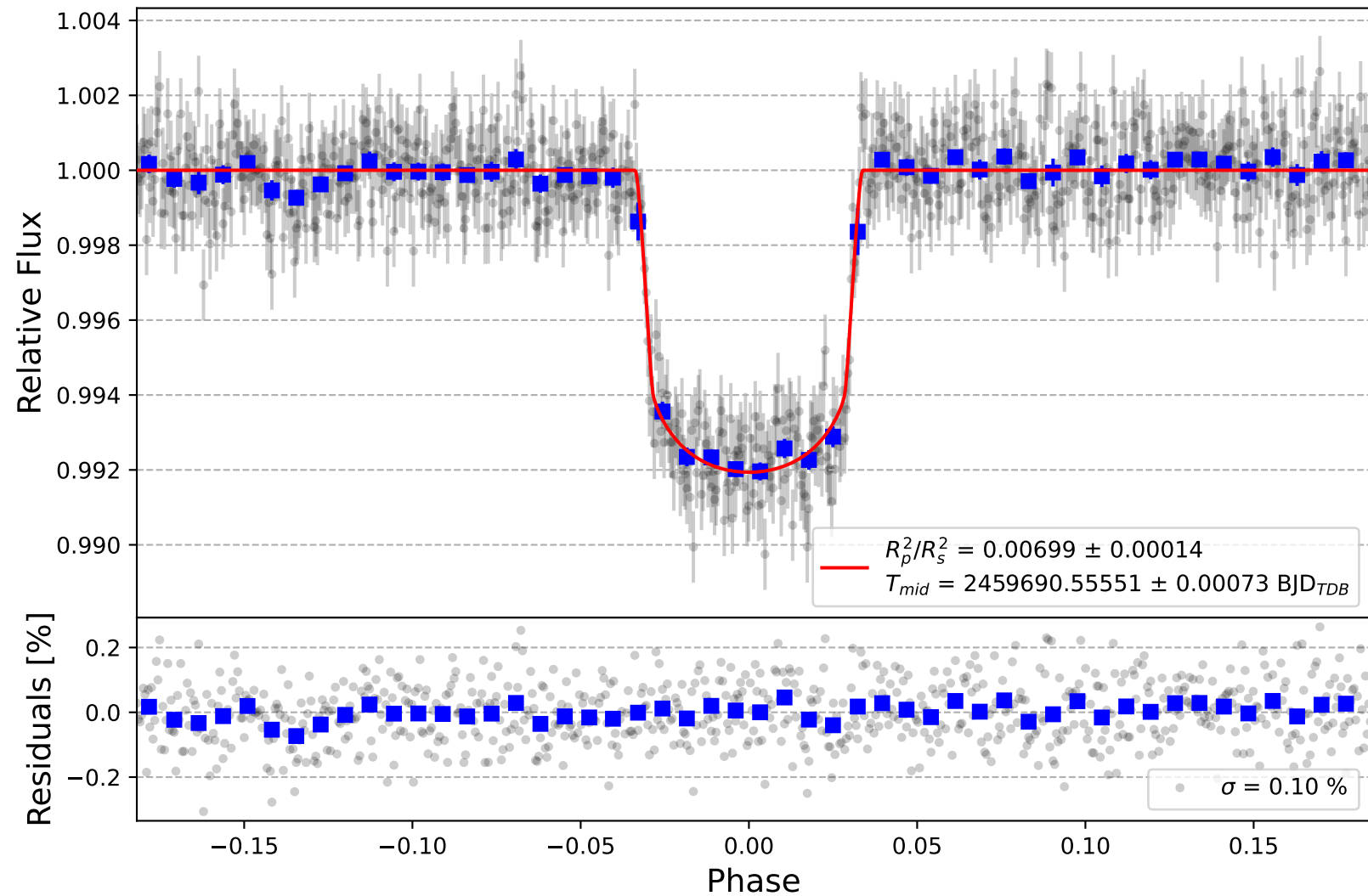
KELT-18 b
