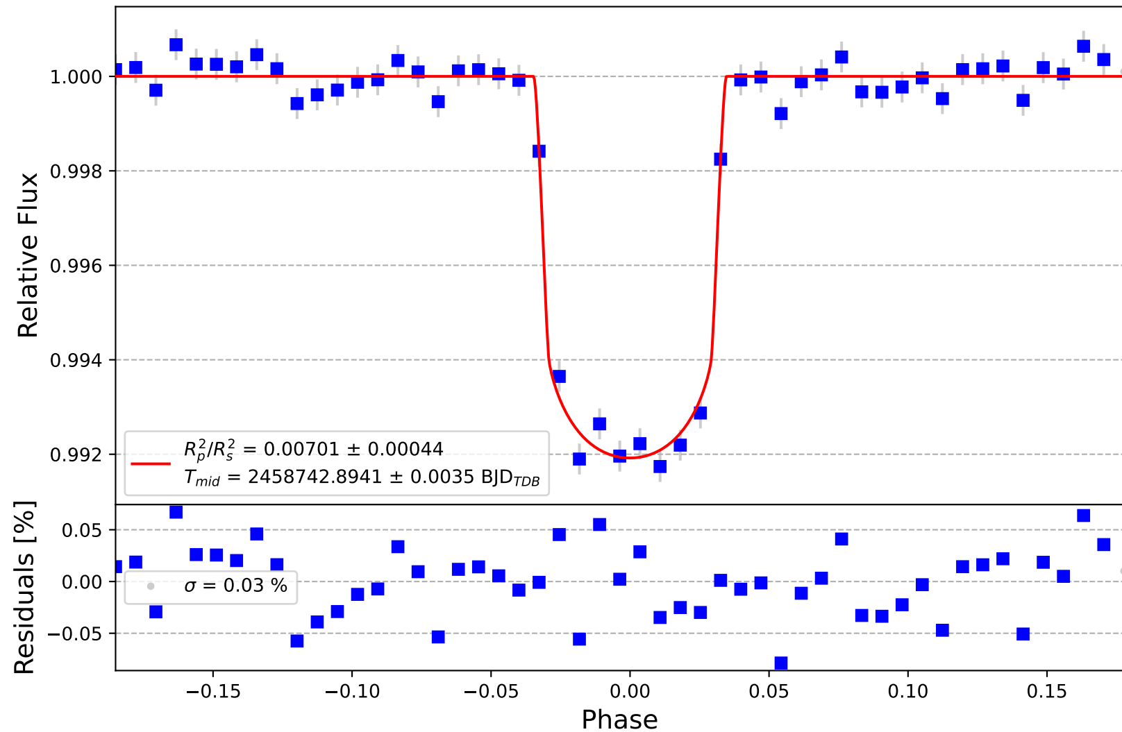
KELT-18 b
