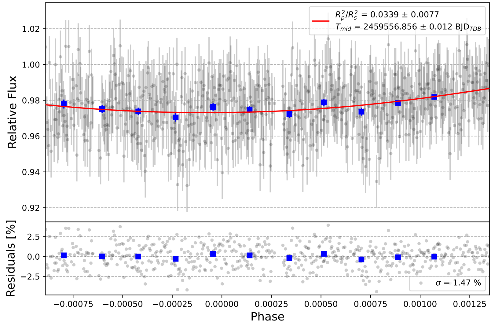
HD 80606 b
