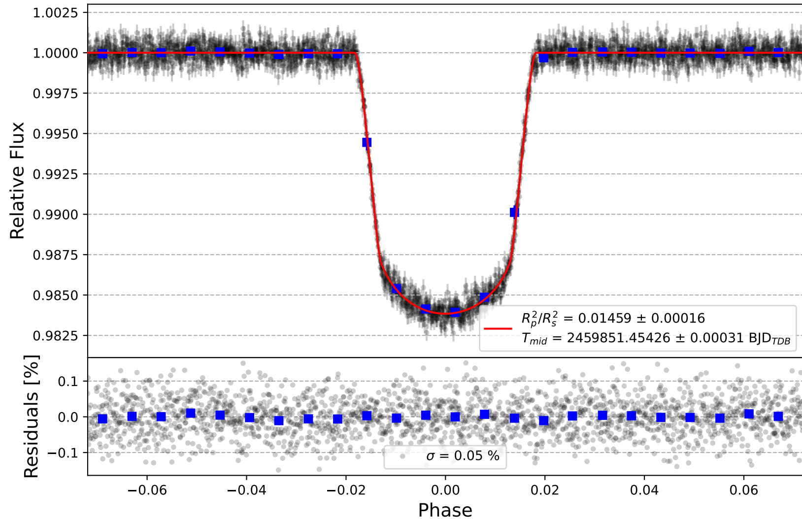
HD 209458 b
