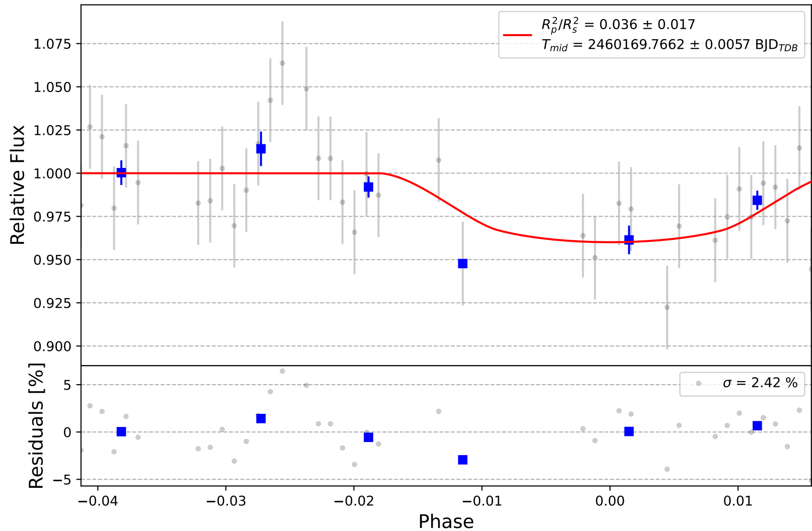
HD 189733 b
