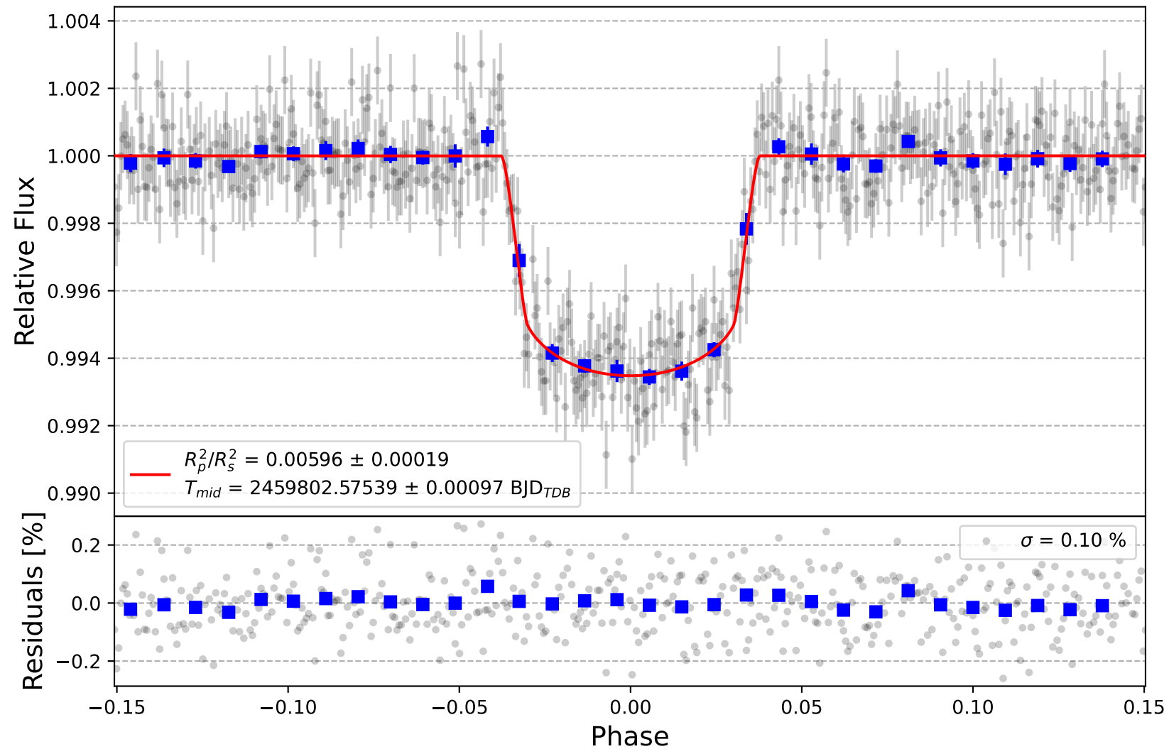
HAT-P-7 b
