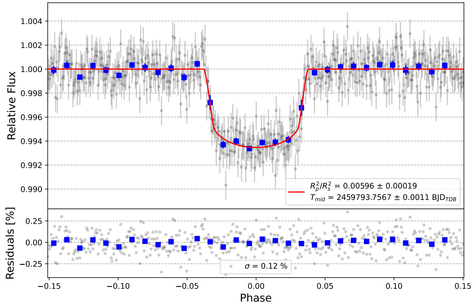
HAT-P-7 b
